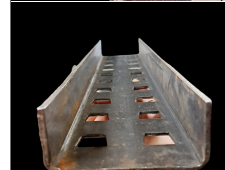
Ceownik perforowany stal czarna 40x80x40x2mm
